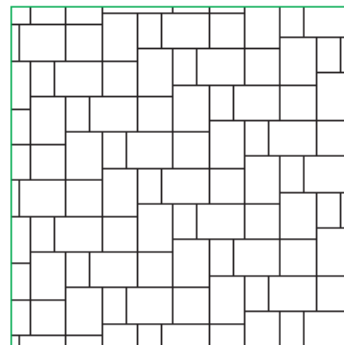
VM 44 - Liana, Rivera, Rustana Bedarf: 21x28 = 10,51 Stk/m 2 21x21 = 5,26 Stk/m 2 21x14 = 5,26 Stk/m 2
