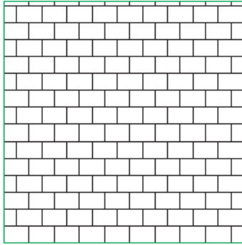
VM 01 - Liana, Rivera, Rustana Bedarf: 14x21 = 34,22 Stk/m 2
