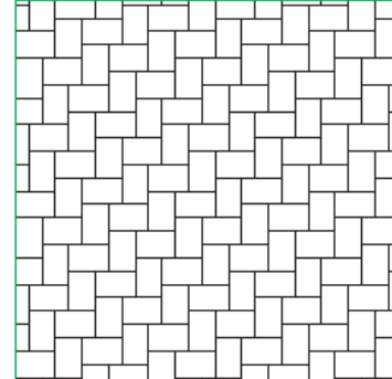
VM 24 - Liana, Rivera, Rustana Bedarf: 21x14 = 34,22 Stk/m 2
