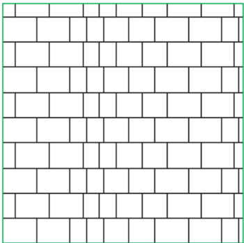
VM 37 - Liana, Rivera, Rustana Bedarf: 21x28 = 7,59 Stk/m 2 21x21 = 7,59 Stk/m 2 21x14 = 7,59 Stk/m 2
