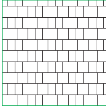
VM 47 - Liana, Rivera, Rustana Bedarf: 21x28 = 6,22 Stk/m 2 21x21 = 6,22 Stk/m 2 21x14 = 12,43 Stk/m 2
