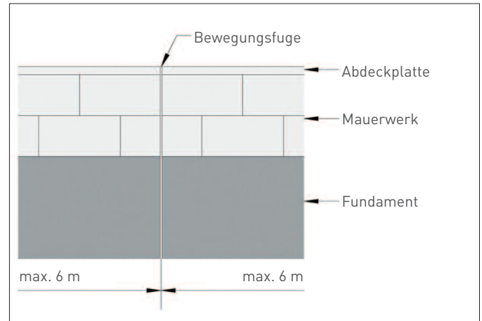
Abbildung 3: Bewegungsfuge
