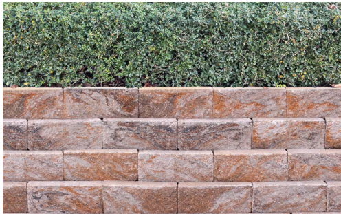
Humuszelle (3D-Symbolbild)
